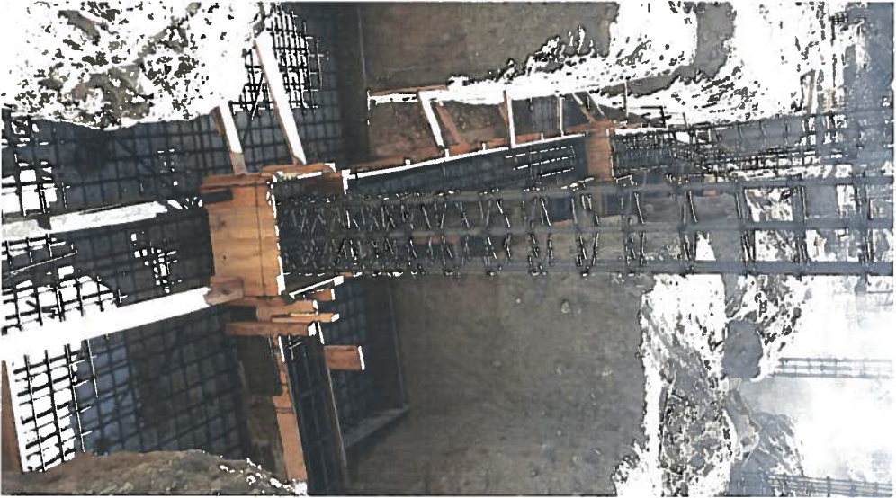
ARMADO Y CIMENTADO DE ZAPATAS AISLADAS
